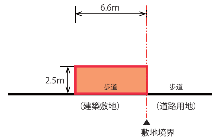
C-C断面
