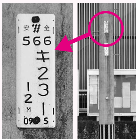
▲写真の電柱番号の読み方
