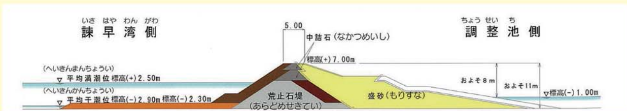
潮受堤防の構造
