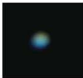
海王星
