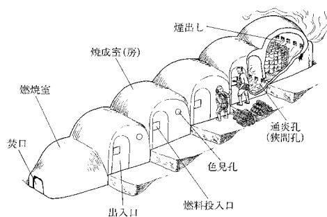
階段式登窯
