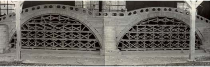
◀完璧な移設復元のために模型実験が必要とされ、石工組合員に模型石製作を依頼し、石材の数も形も全く同じ5分の1スケールの眼鏡橋の模型を造った。
