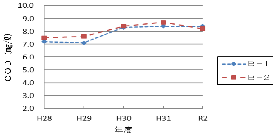
図2-1-4 調整池の水質経年変化 (COD)
