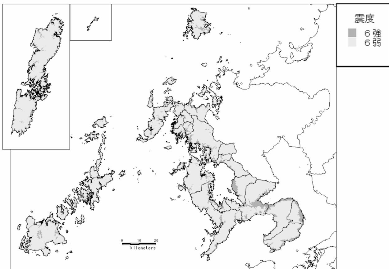
図－１３ 県内全域で M6.9（震源断層上端の深さ 3km）の地震を想定した場合の震度分布
