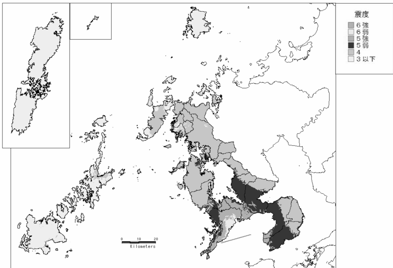
図一 9 地表における推計震度分布（震源：橘湾西部断層帯）
