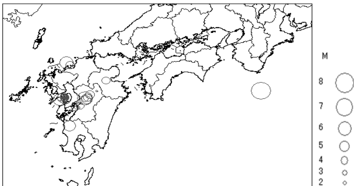
図－2 長崎県内で震度4以上を観測した地震の震央分布図 （1919年～2025年、詳細不明の地震を除く。）長崎地方気象台資料
