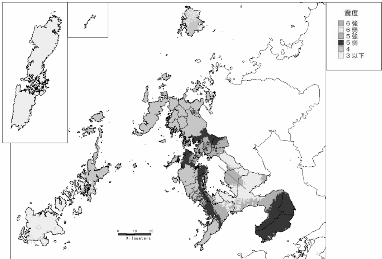
図－１０ 地表における推計震度分布（震源：大村－諫早北西付近断層帯）
