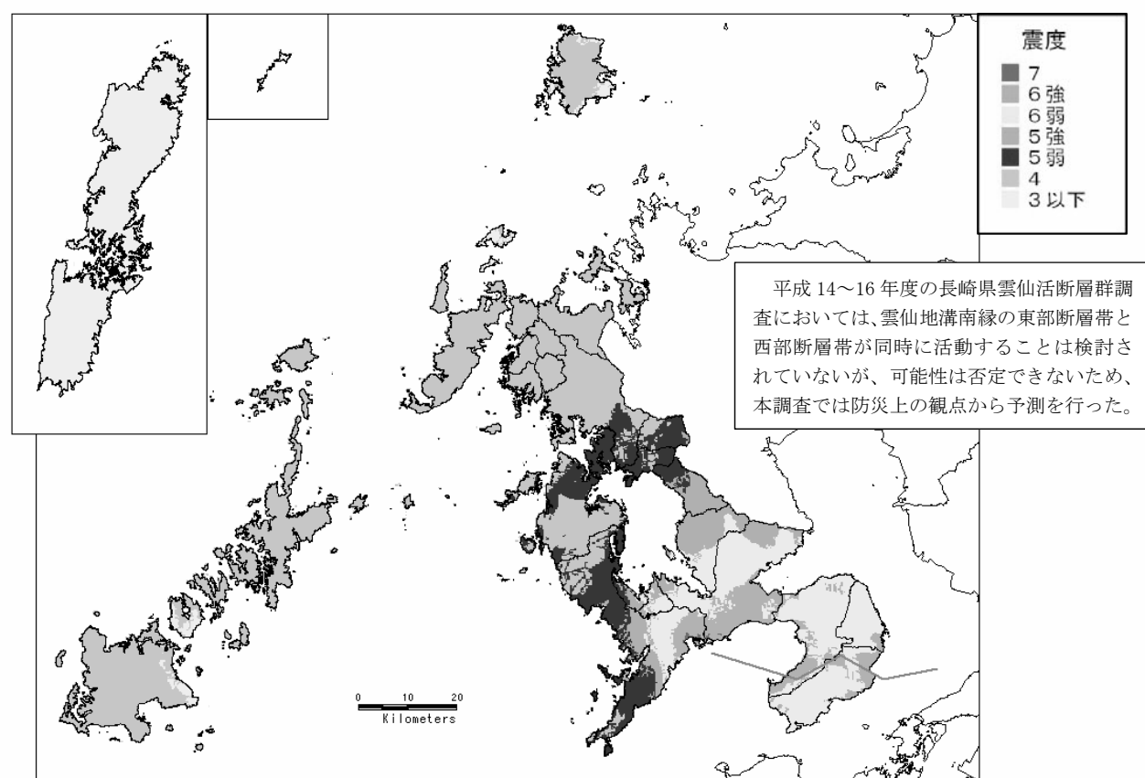
図－５ 地表における推計震度分布（震源：雲仙地溝南縁東部断層帯と西部断層帯の連動）
