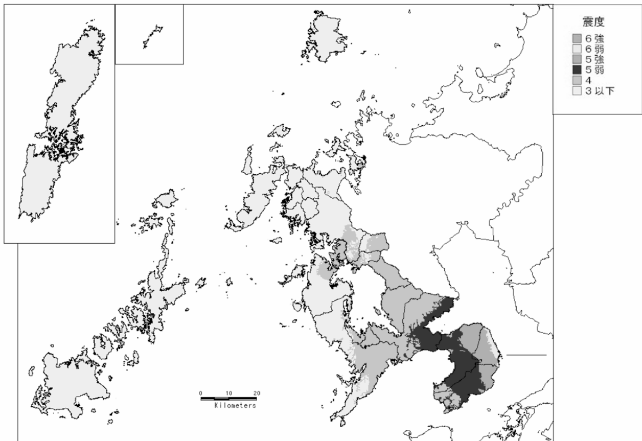
図一 8 地表における推計震度分布（震源：島原沖断層群）
