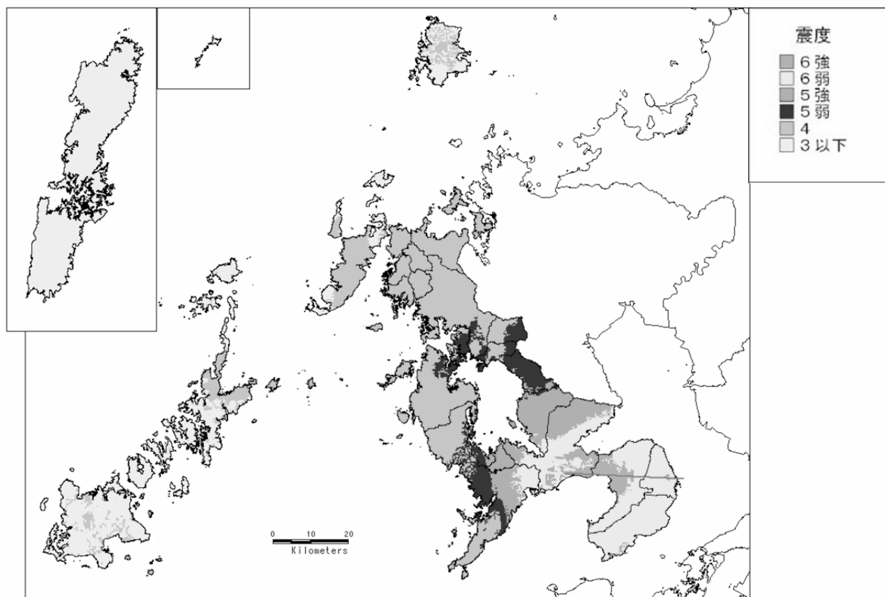
図－４ 地表における推計震度分布（震源：雲仙地溝北縁断層帯）
