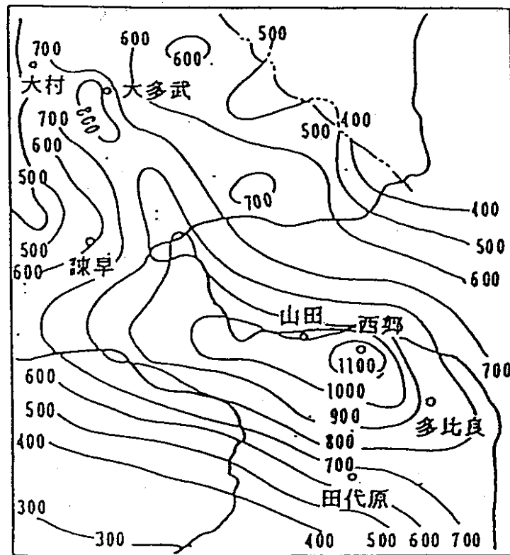
昭和32年7月25日9時～26日9時の降水量分布図
