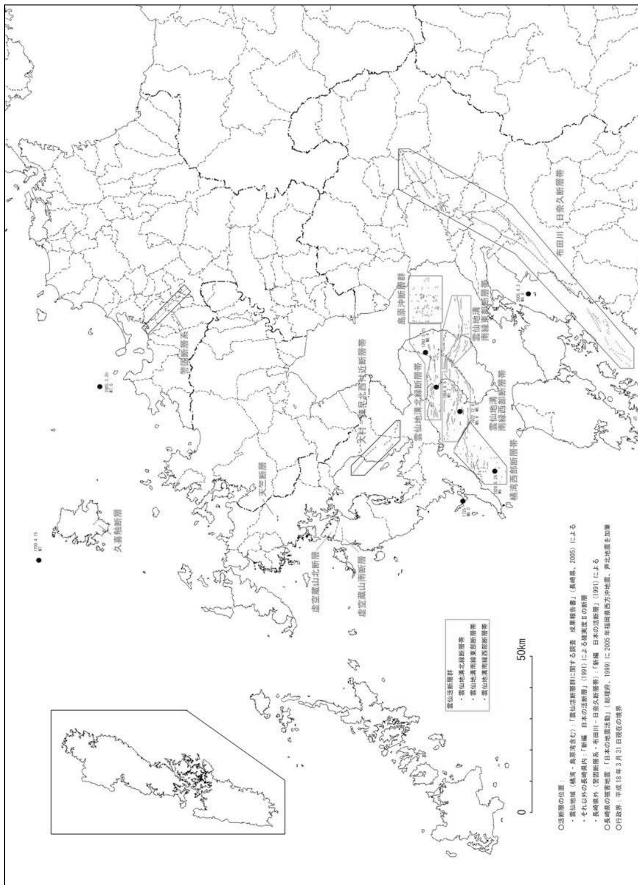
図一3 震源となる活断層の位置図
