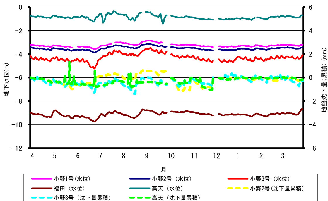
図2-6-7 地下水位と地盤沈下量の変化(令和元年度)
