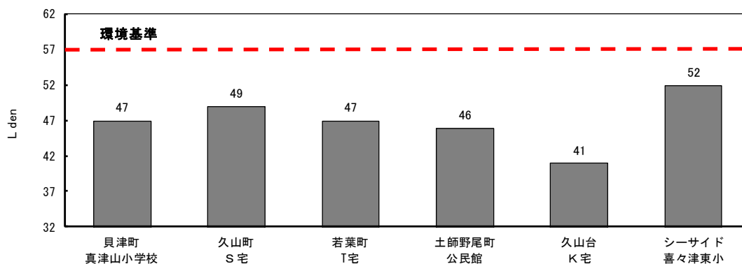
図2-1-7 各測定地点のLden(令和元年度)
