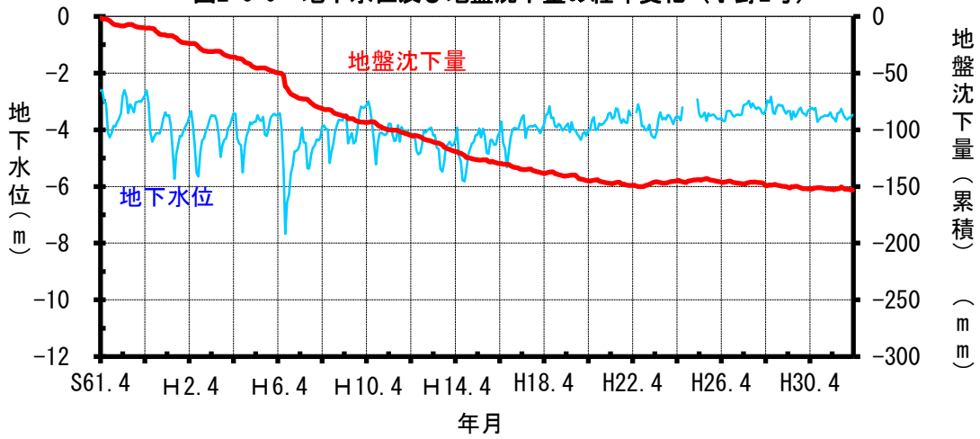
図2-6-9 地下水位及び地盤沈下量の経年変化（小野2号）
