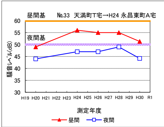
図2-1-6 環境騒音の経年変化
