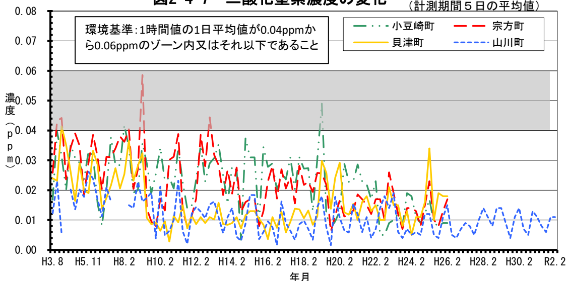
図2-4-7 二酸化窒素濃度の変化 (計測期間5日の平均値)
