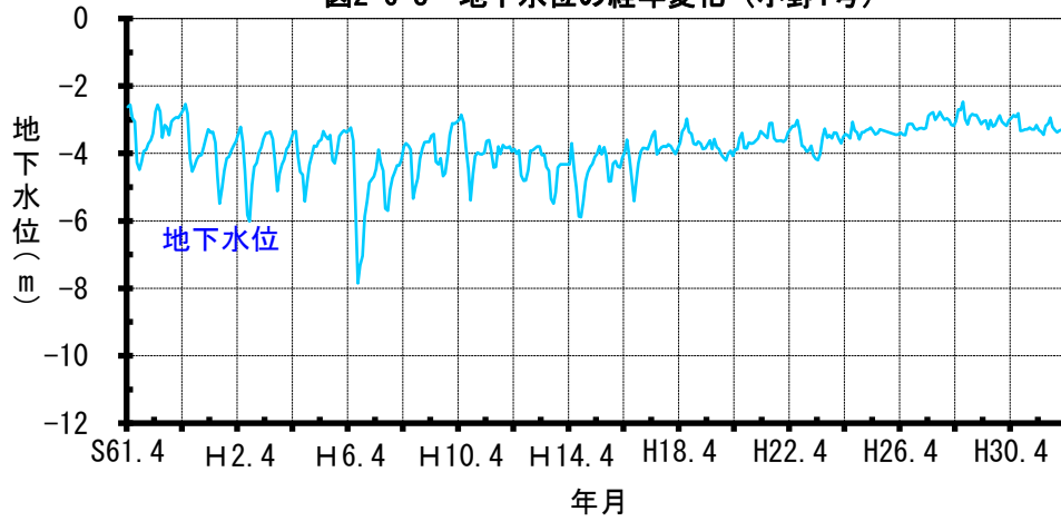
図2-6-8 地下水位の経年変化（小野1号）
