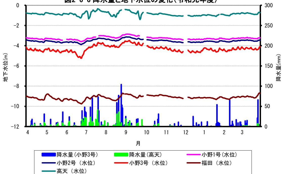
図2-6-6 降水量と地下水位の変化(令和元年度)
